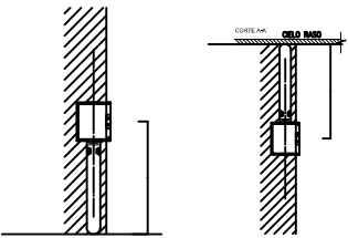
DETALLES TOMACORRIENTE
