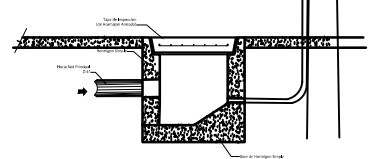
DETALLES PARA ACOMETIDA MEDIA TENSION
