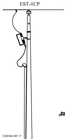
DETALLES ACOMETIDA EN BAJA TENSION Y CAJA DE REVISION
