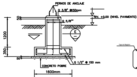
FUNDICIÓN PARA MASTIL EN TIERRA FIRME
