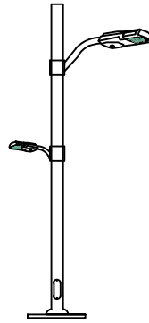
POSTE METALICO 3-4 M DOBLE LAMPARA DISTINTO W
