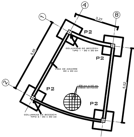
PLANTA DE CIMENTACION ESC: 1:50
