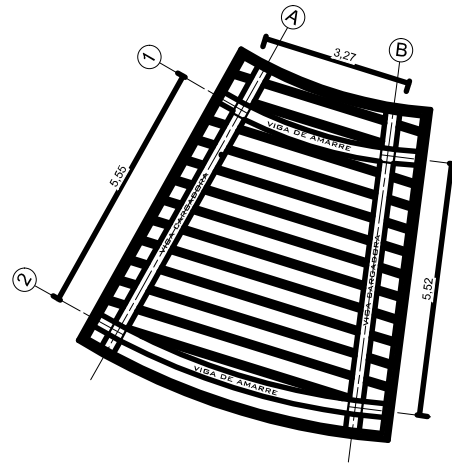
ARMADO DE LOSA TIPO N+3.00 ESC: 1:50
