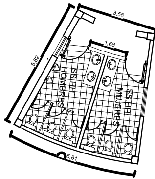
PLANTA DE BAÑOS AREA DE GIMNASIA ESC: 1:50
