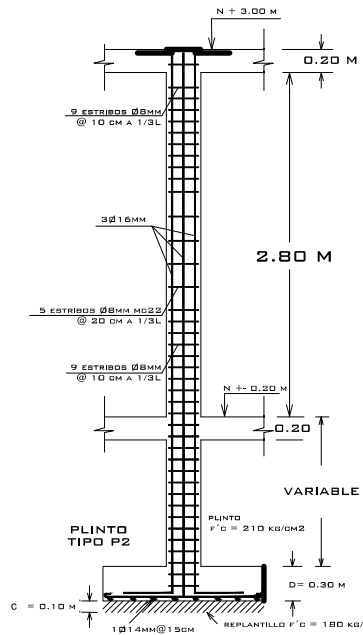
DETALLE DE COLUMNA Y PLINTO ARMADURA ESC: 1:20
